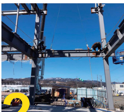
鉄骨建方
